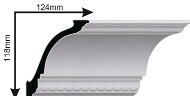
VD22G (118/124 mm x 2 m) - Skin-Tec
